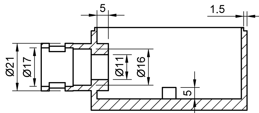
A-A (1:1)
